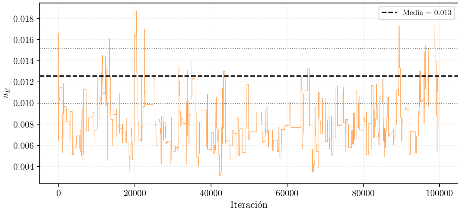
Cadena MCMC - u_E
